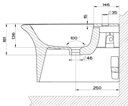
SEZIONE A-A
