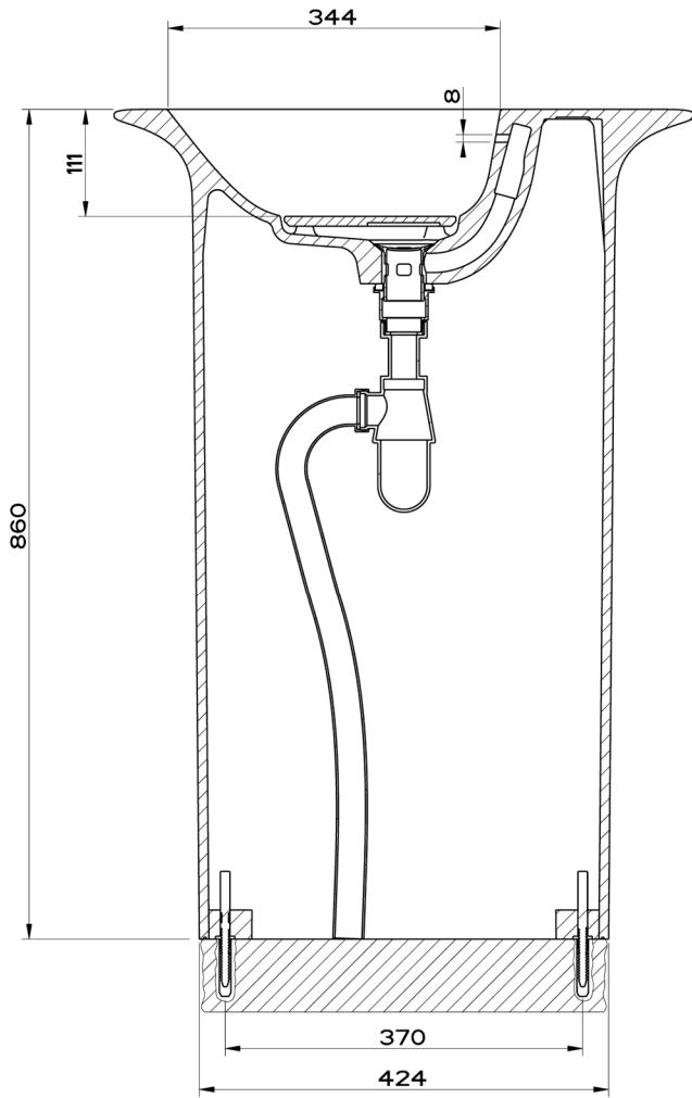
SEZIONE A-A
