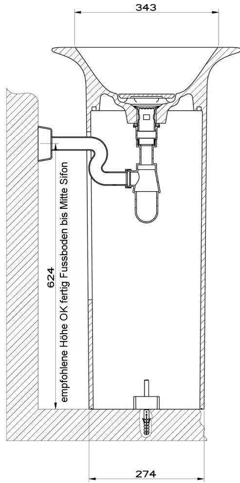
SEZIONE B-B
