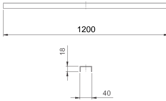
Abdeckung Standard
