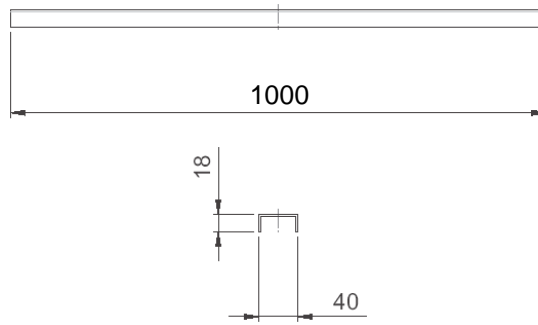
Abdeckung Standard
